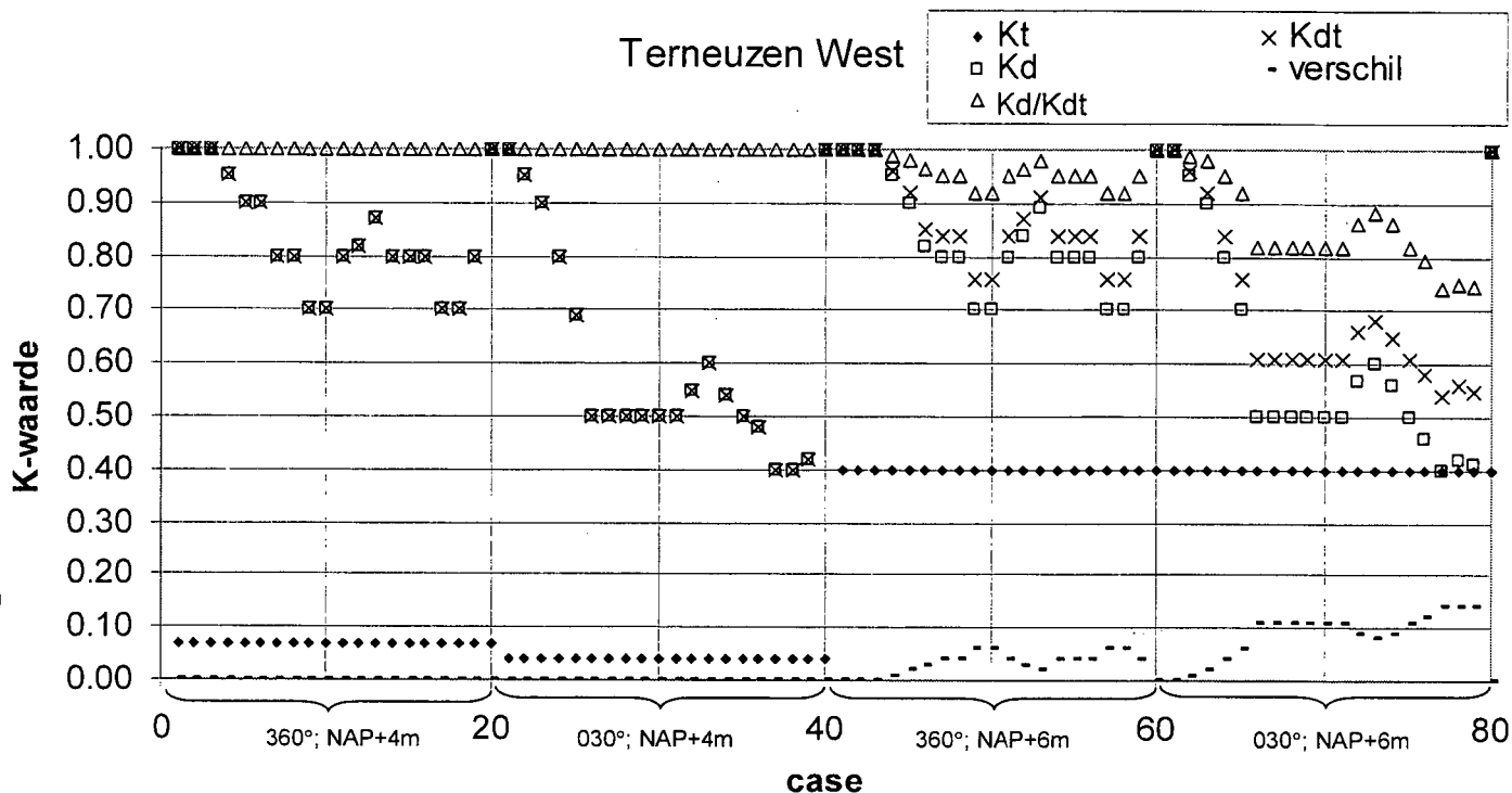
Bijlage 3.8.a: Kt, Kd, Kdt en verschil voor Terneuzen West. Linkerheft: NAP+ 4m; Rechterheft: NAP + 6 m Telkens 20 uitvoerpunten op een rij, te weten locaties 1 t/m 20
