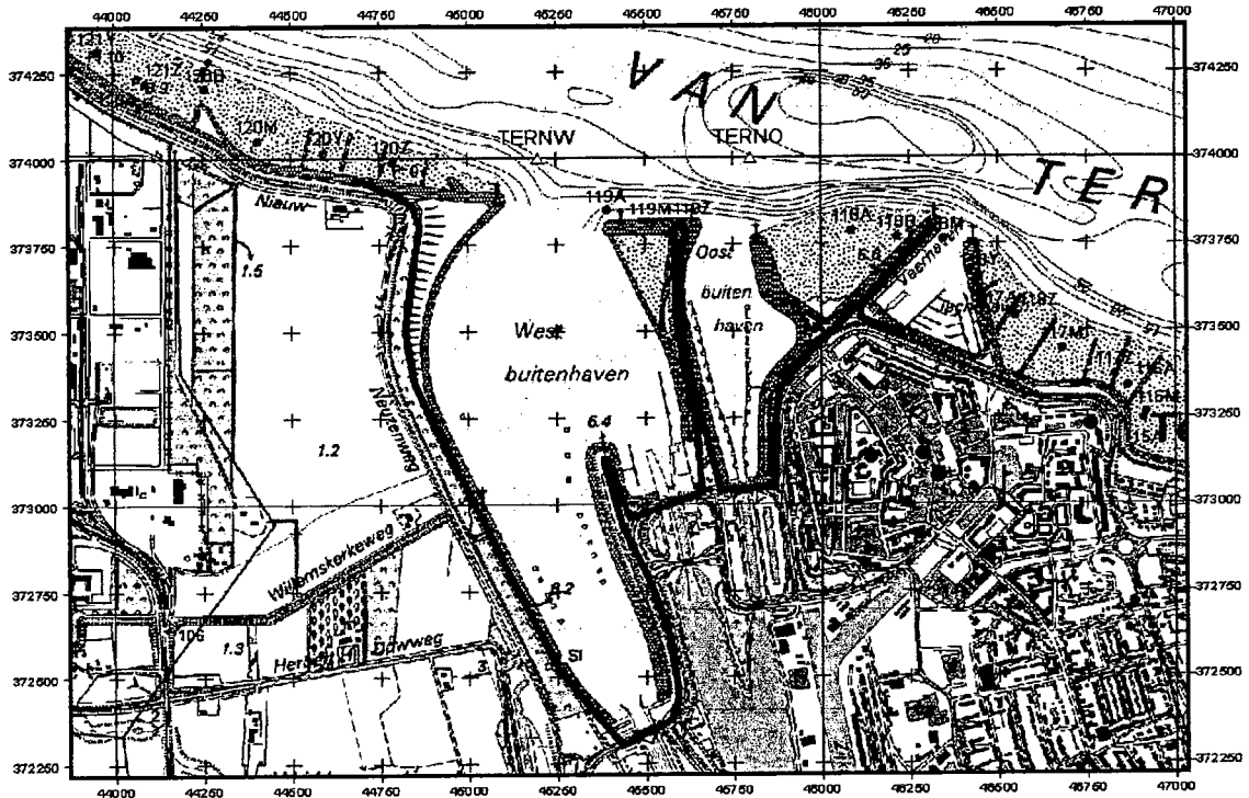
Fig 1.1: Topografie Westbuitenhaven, Oostbuitenhaven en Scheidingsdam Terneuzen ——— primaire zaewering
