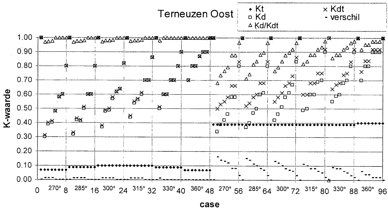
Bijlage 3.8.b: Kt, Kd, Kdt en verschil voor Terneuzen Oost. Linkerheft: NAP+ 4m; Rechterheft: NAP + 6 m Telkens 8 uitvoerpunten op een rij, te weten locaties 21 t/m 28
