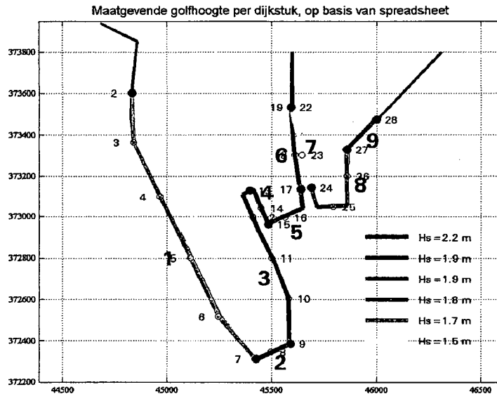
Figuur 3.2: Maatgevend Hs per dijkstuk bij NAP +6m op basis van spreadsheetmethode
