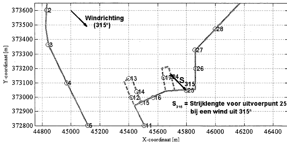
Figuur 3.3: Schematisatie situatie zonder scheidingsdam.
