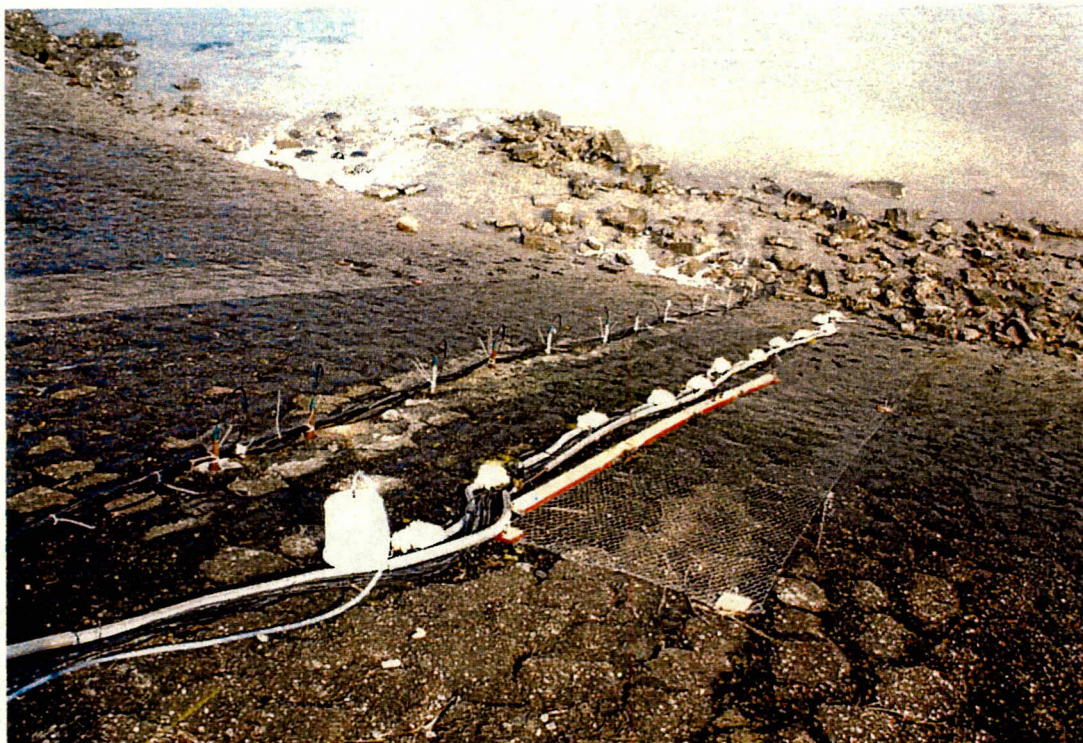
Foto, Meetopstelling Baarland
