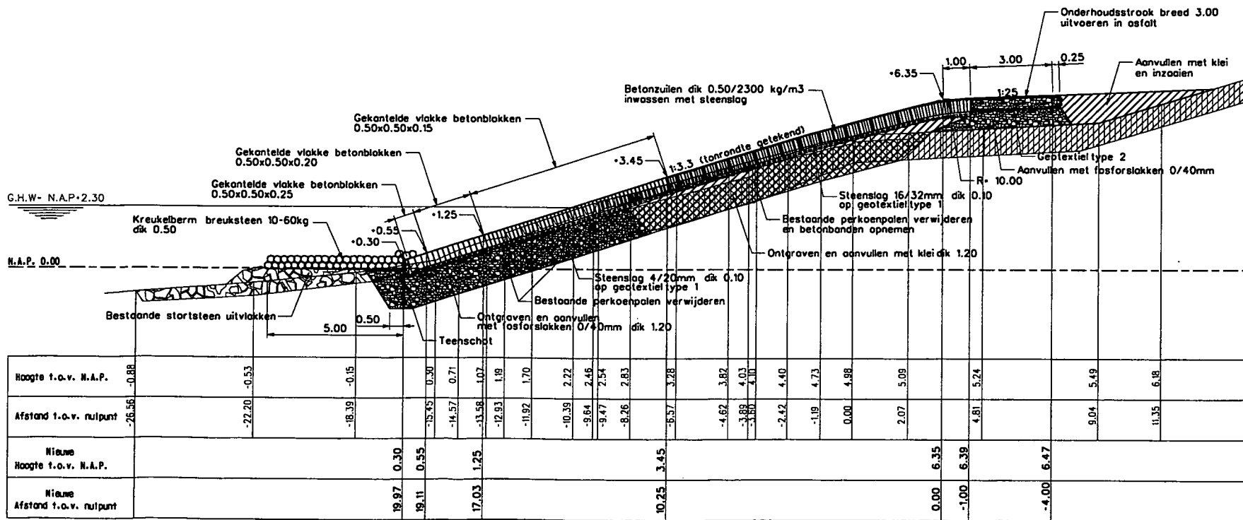
Dwarsprofiel 2 nieuw
