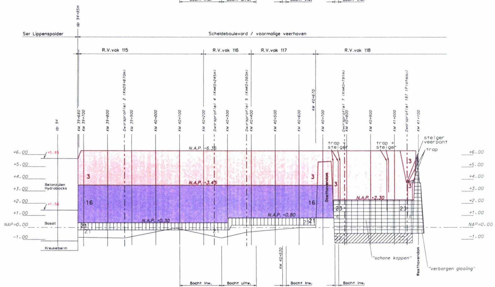
Glooiingskaart alternatief 3
