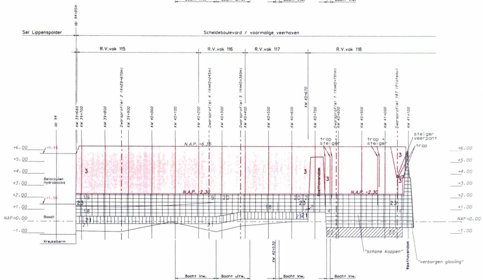
Glooiingskaart alternatief 2
