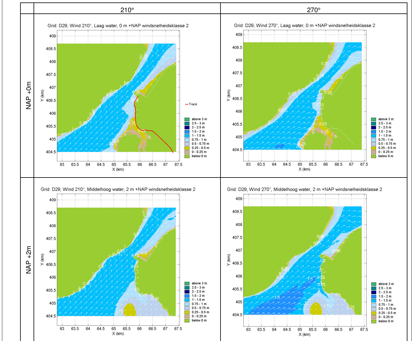
Figuur 4 toont de met SWAN berekende golfhoogte H_s (zonder enige correcties) voor de windrichting 210 - 270° bij de waterstanden NAP +0m, +2m en +4m. Duidelijk zichtbaar is dat het slik bij een waterstand van NAP +4m minder invloed heeft op de golfcondities. Er is in die situatie voldoende waterdiepte beschikbaar, waardoor het slik vrijwel niet golfreducerend werkt.
