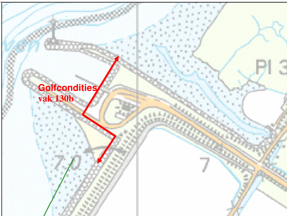
Figuur 3: Aanpassing dijkvakken t.p.v. veerhaven
