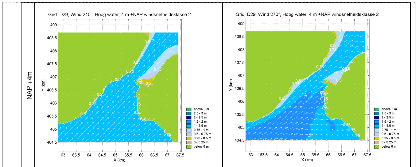
Figuur 4: SWAN resultaten voor H_s . Van links naar rechts met ruimende wind, van boven naar onder met toenemend waterpeil.
