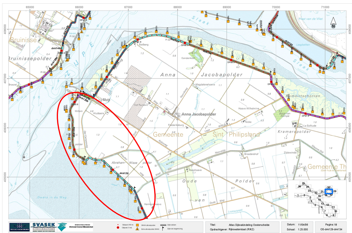
Figuur 2: Dijkvakken 128 t/m 130b
