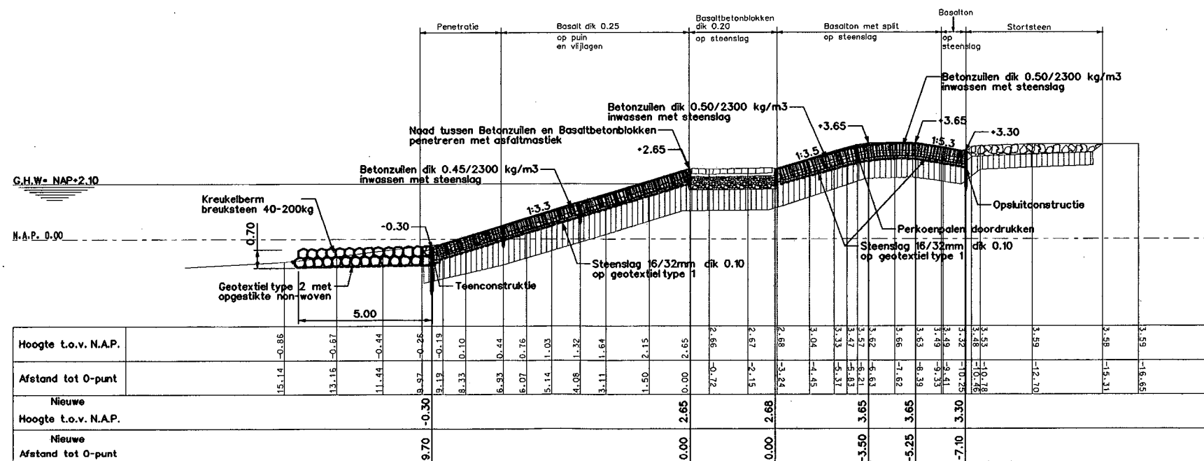
Dwarsprofiel 10 nieuw
